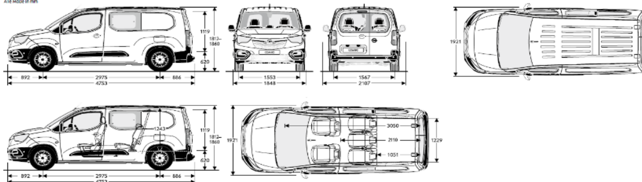
Combo Doppelkabine Alle Maße in mm
